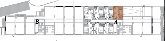
TLOCRT PRIZEMLJA
